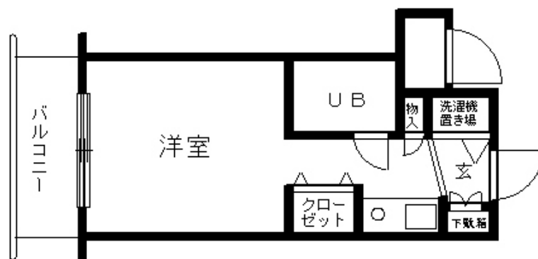
【間取り図】
