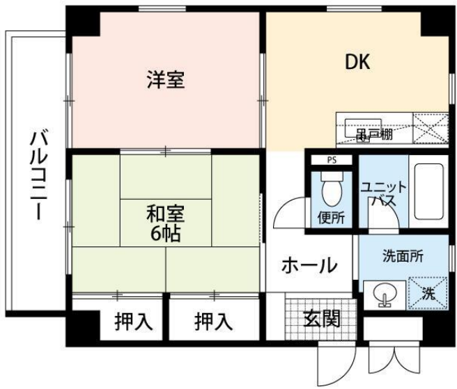
【間取り図】
